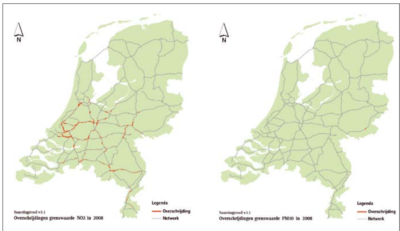
Figuur 5.8 Overschrijdingen langs het HWN in 2008 voor de daggemiddelde grenswaarde \text{PM}_{10} (links), en de jaargemiddelde grenswaarde voor \text{NO}_2 (rechts)
