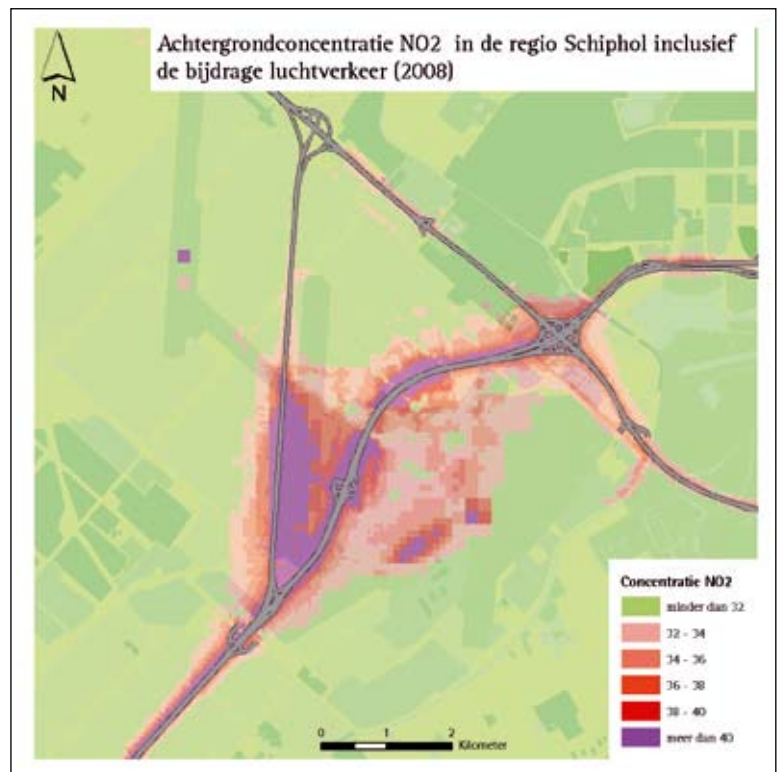
Figuur 5.7 Achtergrondconcentratie \text{NO}_2 in 2008 plus de bijdrage van de luchtvaart rond Schiphol ( \mu\text{g}/\text{m}^3 ) 69
